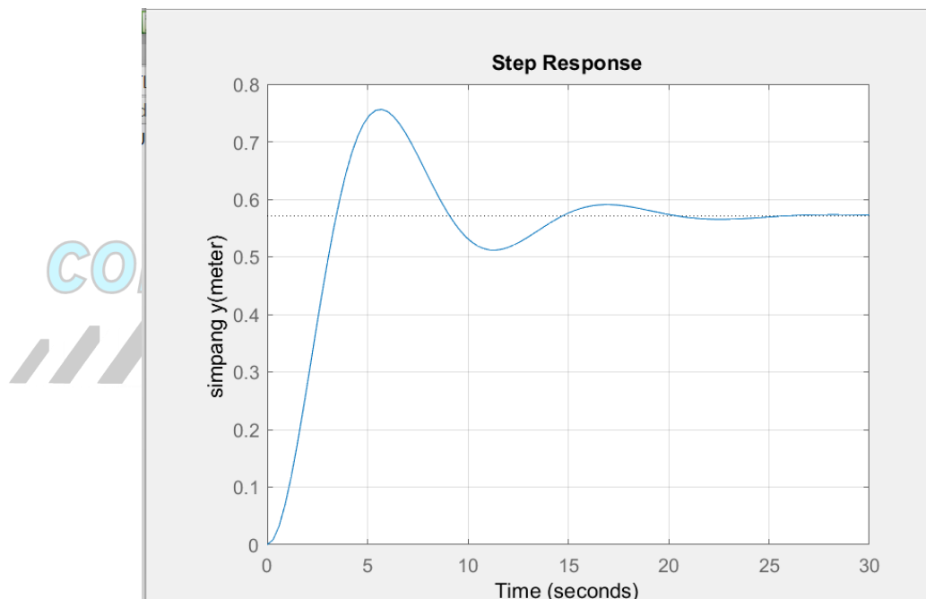
Gambar 3. 2 Kurva Keluaran Step Sistem Orde 2
