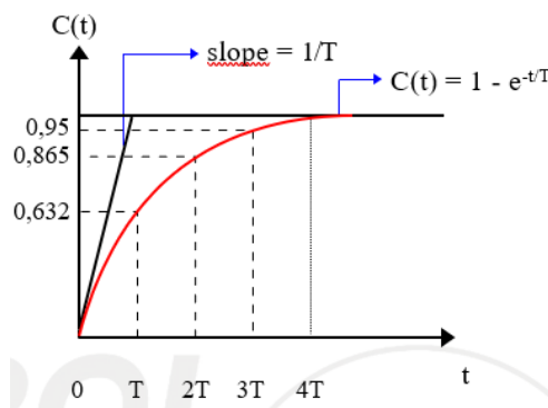
Gambar 2. 1 Respons Unit Step Sistem Orde Satu
