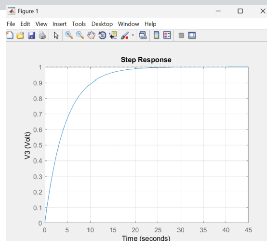
Gambar 2. 2 Respons Unit Step Sistem Orde Satu.
